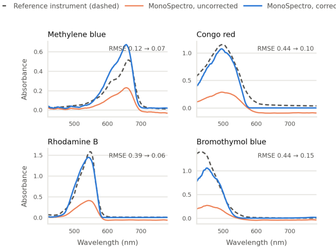
Fig. 3. El conjunto de test: cuatro colorantes de laboratorio medidos en una sesión posterior, mostrados sin corregir, corregidos y tal como los registra el instrumento de referencia (línea discontinua).
