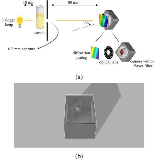
Fig. 1. (a) Camino óptico. La luz de la fuente halógena atraviesa la cubeta y la rendija de entrada y la dispersa una red de difracción pegada directamente a la cara frontal de la lente, sobre un sensor inclinado 36^\circ . (b) El instrumento montado. [sustituir por la fotografía principal de la unidad construida]
