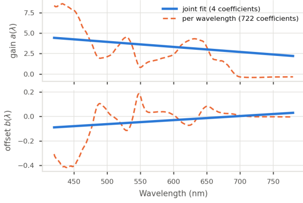
Fig. 2. La corrección ajustada. El ajuste por longitud de onda es libre de seguir a las muestras de entrenamiento, mientras que el ajuste conjunto de primer grado son dos rectas. El modelo restringido conserva la deriva y elimina las excusiones.
